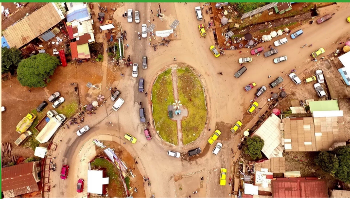
Levé topographique du Rond point Tannerie avec prises de vue aérienne
